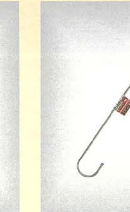
SBH450 18-8ステンレスS型玉付フック450mm ①A: 450 B: 52 C: 52 ②5.0φ ③本体巻シール ④20/120入 ⑤5kg ⑥4530770440363 ⑦玉付
