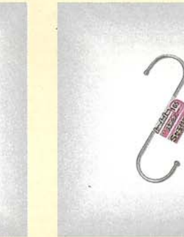
SBH165 18-8ステンレスS型玉付フック165mm ①A: 165 B: 40 C: 40 ②5.0φ ③本体巻シール ④20/240入 ⑤5kg ⑥4530770440165 ⑦玉付
